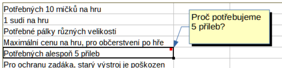
Obrázek 419: Prohlížení komentáře
