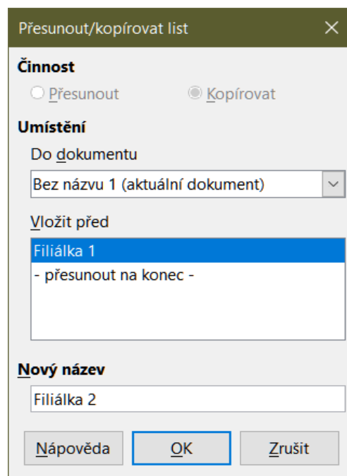
Obrázek 228: Kopírování listu
