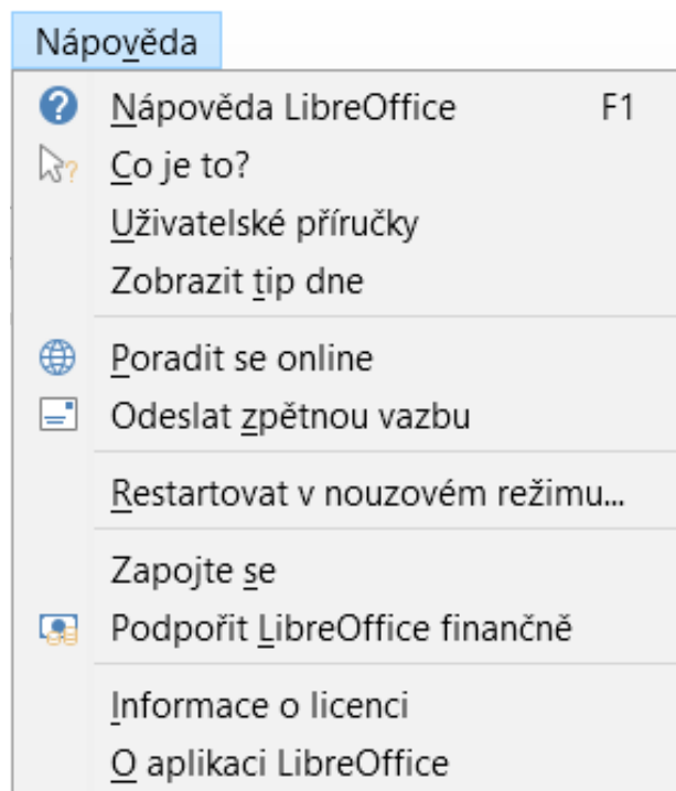
Obrázek 1: Nabídka nápověda
