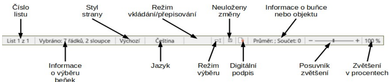
Obrázek 5: Stavový řádek
