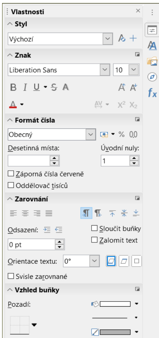
Obrázek 6: Postranní lišta
