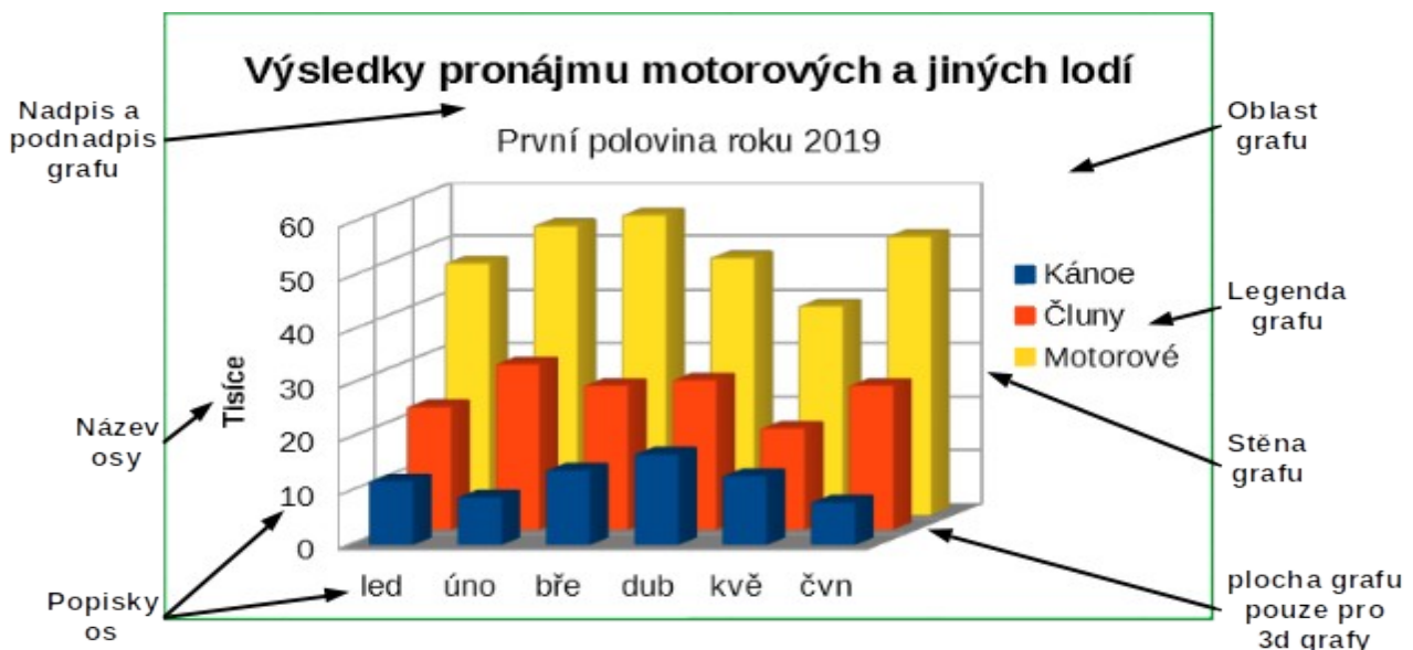
Obrázek 78: Prvky grafu
