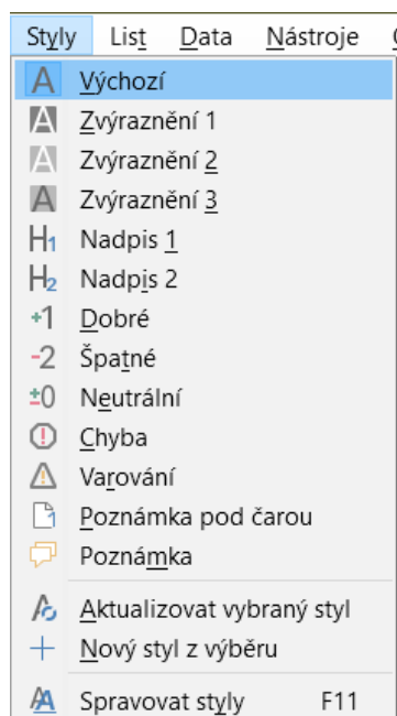
Obrázek 156: Nabídka stylů
