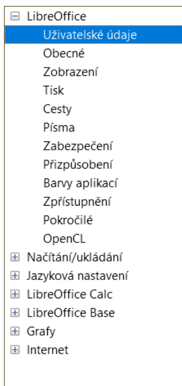
Obrázek 473: Možnosti LibreOffice
