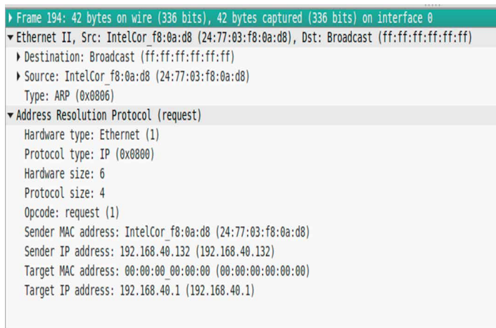
Obrázek 50: Paket ARP protokolu zachycený programem Wireshark
