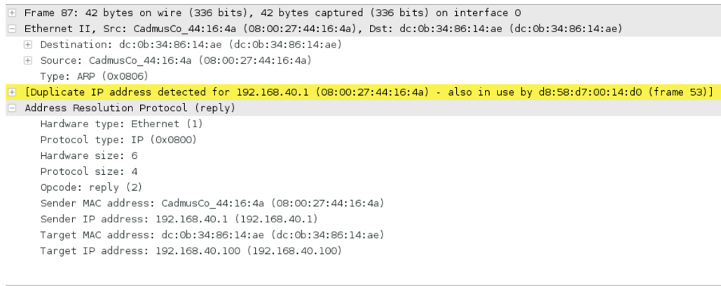
Obrázek 53: ARP Cache poisoning zachycený programem Wireshark. Ten umí na případnou duplikaci MAC adres upozornit.
