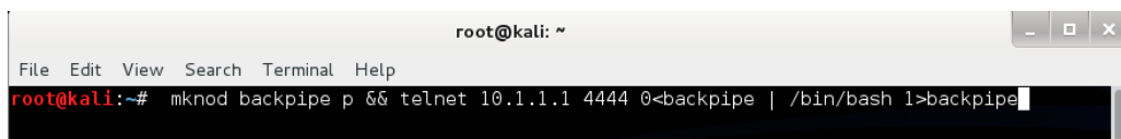
Obrázek 47: Ukázka kódu otevírajícího reverzní shell vloženého Teensy - zde je vše záměrně dobře viditelné
