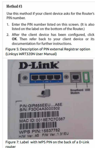
Obrázek 59: WPS PIN 503
