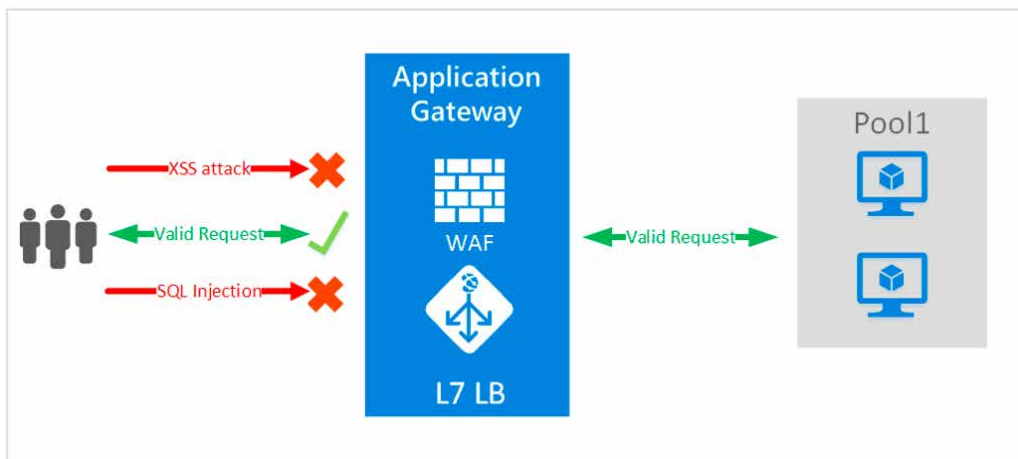
Obrázek 61: Aplikační gateway 522
