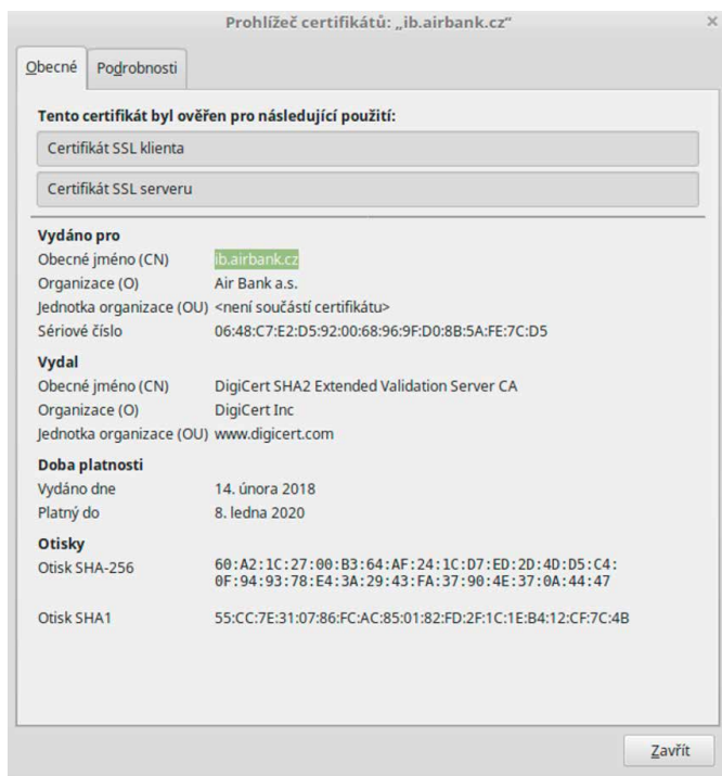
Obrázek 69: Pravý certifikát
