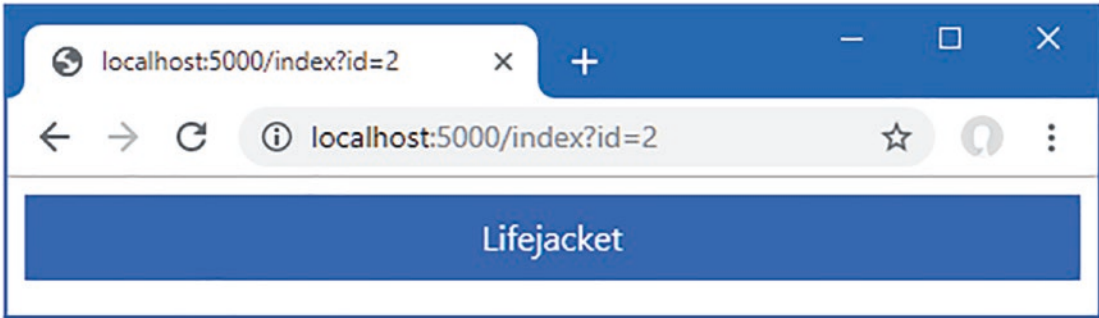
Figure 23-5. Using a query string parameter
